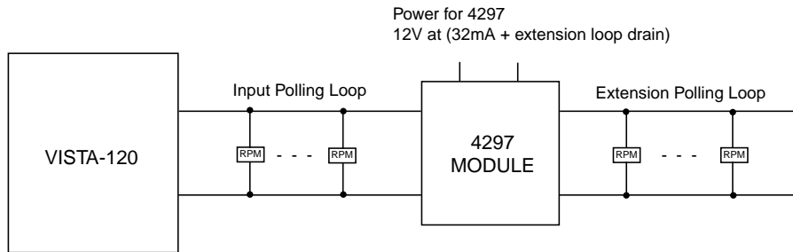
图 13a. 使用一个 4297 模块的总线连接
