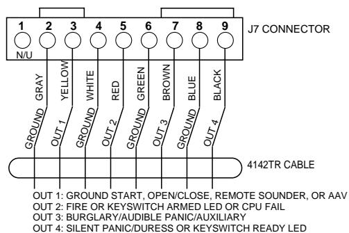
图 20: J7 触发器
