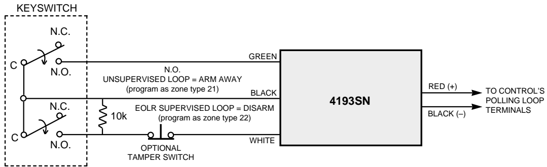
图 23b. 分子系统配置布撤防锁
