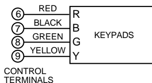
图 6. 键盘和主机间的连接
