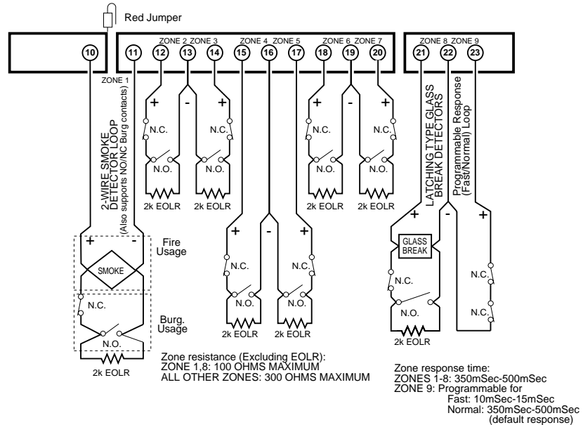
图 8: 防区 1-9 连线图
