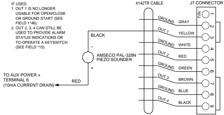
图 22. 键盘发声器连接
